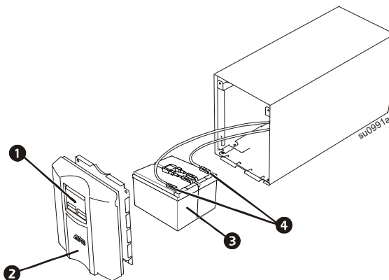
SMT2200C, SMT2200IC, SMT3000C och SMT3000IC Tower
