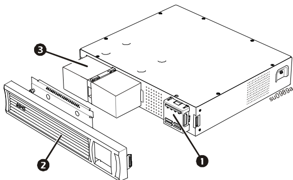
SMT1000RM2UC, SMT1000RM12UC, SMT1500RM2UC och SMT1500RM12UC rackmonterad
