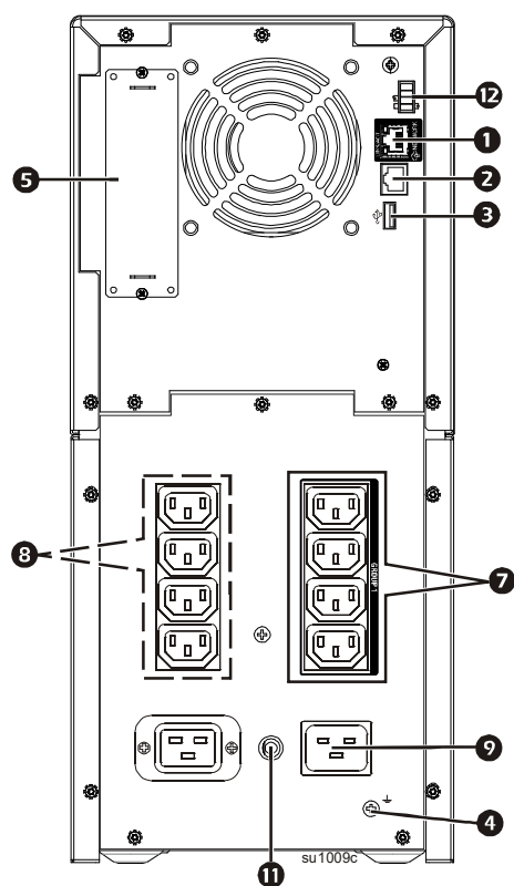
SMT2200IC och SMT3000IC Tower
