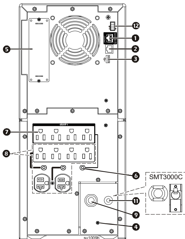
SMT2200C och SMT3000C Tower
